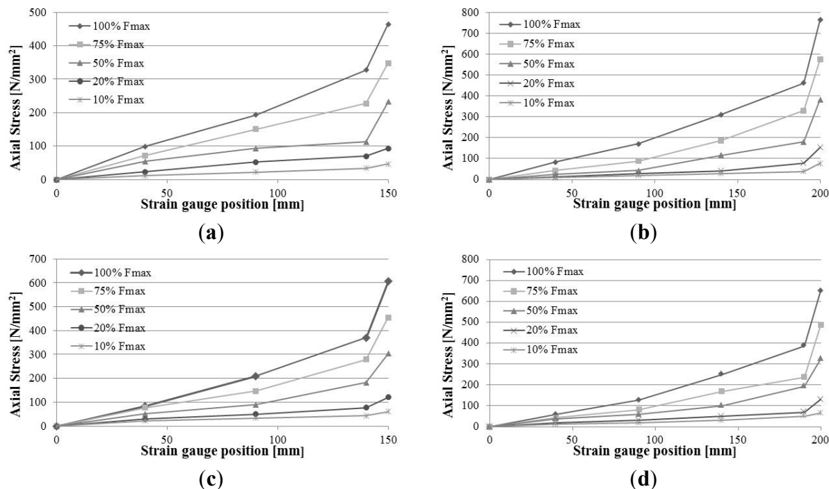
Figure 12. Normal stress versus position: (a) SF_2 test; (b) SF_4 test; (c) SC_2 test; (d) SC_4.
