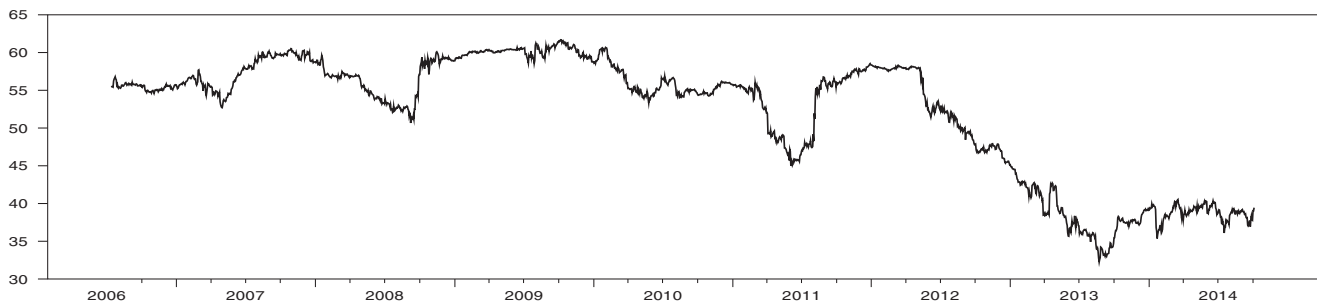
Fig. 5. Intra-regional return spillovers plot.
