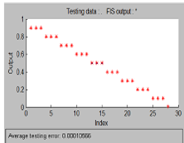
Fig. 7. Test result
